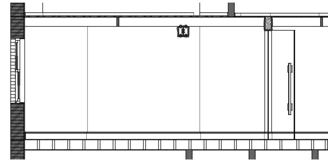
Elevation 4
