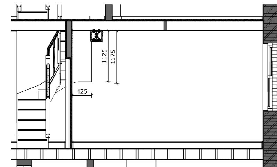
Elevation K1
