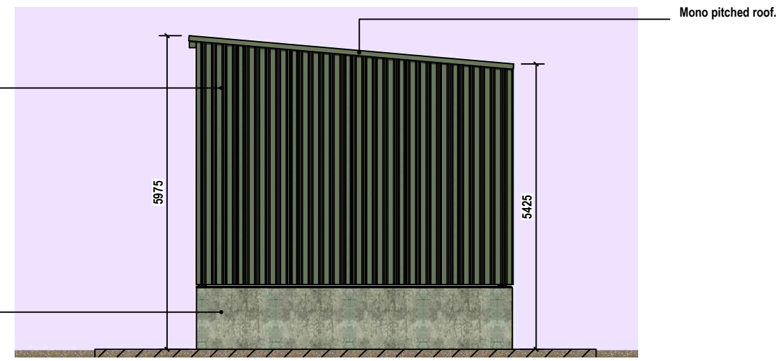
Elevation - side 1 (RI) Scale: 1/100
